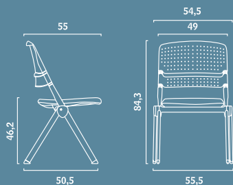
8DRF100P schienale fisso 8DRR100P schienale oscillante
