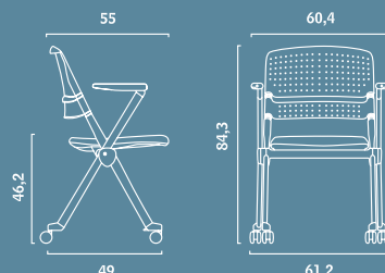
8DRR500R 1 bracciolo/schienale fisso 8DRF200R 2 braccioli/schienale fisso 8DRR500R 1 bracciolo/schienale oscillante 8DRF200R 2 braccioli/schienale oscillante
